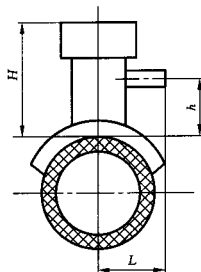
图 2 管件承口端示意图
